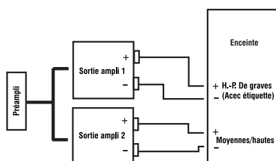
Figure 2 : Raccordement et amplification à sources multiples entre les enceintes et l'amplificateur
