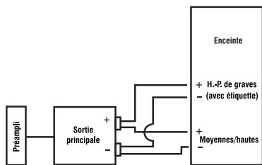
Figure 2 : Raccordement et amplification à sources multiples entre les enceintes et l'amplificateur
