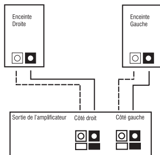
Figure 1 : Câblage en phase entre les enceintes et l'amplificateur
