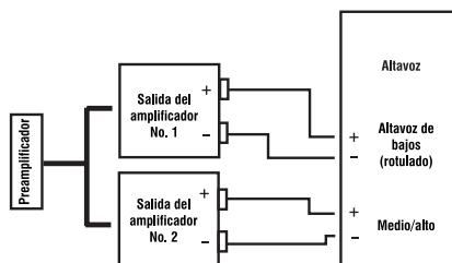
Figura 2: Conexión de doble cableado y de doble amplificador, entre los altavoces y el amplificador
