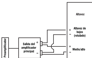
Figura 2: Conexión de doble cableado y de doble amplificador, entre los altavoces y el amplificador
