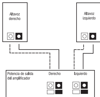
Figura 1: Cableado en fase entre los altavoces y el amplificador
